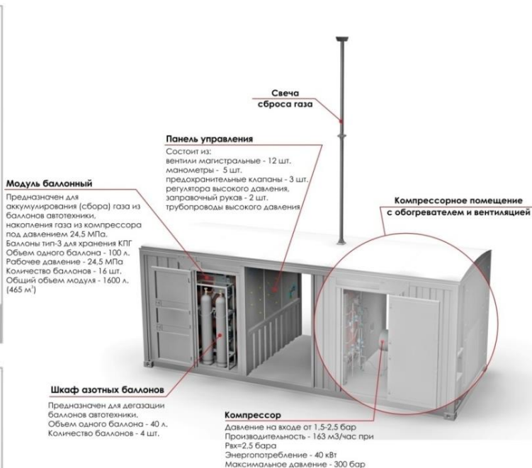
Стенд проверки ГБО и дегазации
